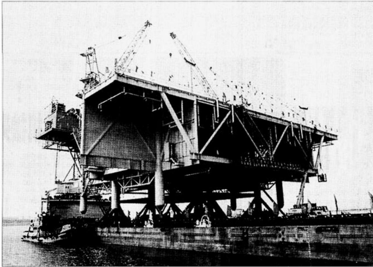
8月28日上午10时30分，由胜利油田有限公司承建的我国目前规模最大的浅海石油开发装备——EDC埕岛西DPA中心平台下水剪彩仪式在油田有限公司海洋工程建造基地隆重举行，这标志着中美合作勘探的渤海埕岛西石油区块正式投入规模开发。
